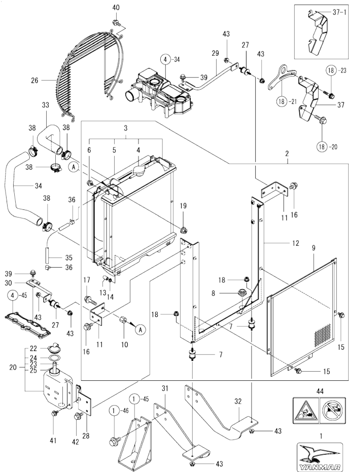
Fig.11. RADIATOR
